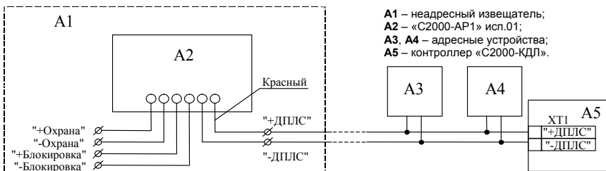
Рисунок 1 Схема соединений
