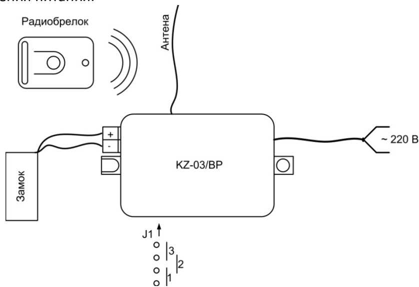
Рис.2. Подключение контроллера к замку
