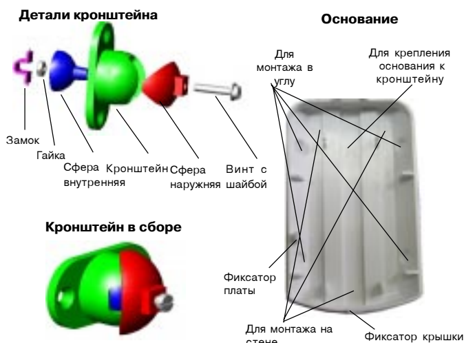
Рис. 3. Основание извещателя и кронштейн
