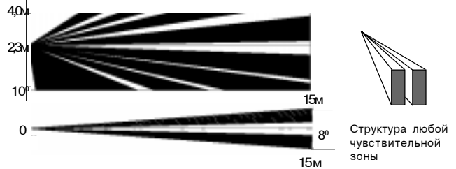
Рис.2 Диаграмма зоны обнаружения извещателя «Фотон-12Б-РК»
